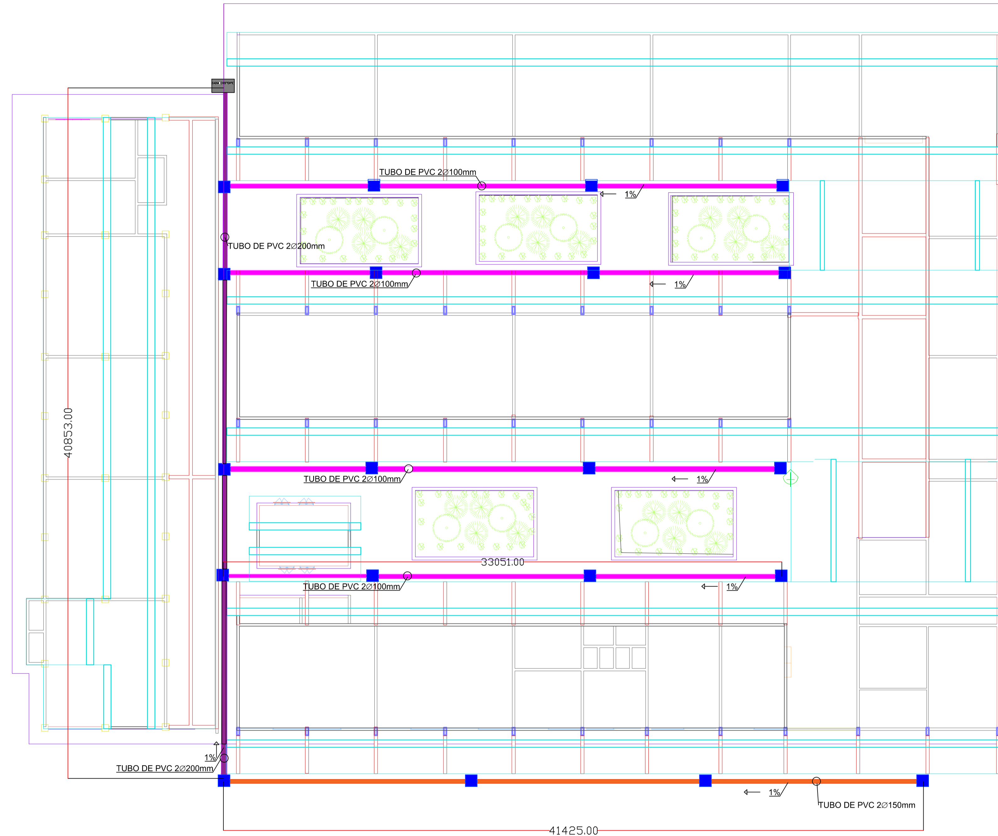
PLANTA PLUVIAL ESCALA 1: 1
